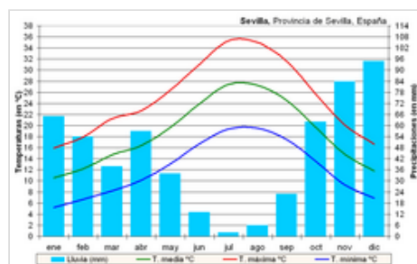
Climograma de Sevilla: datos del observatorio del aeropuerto
